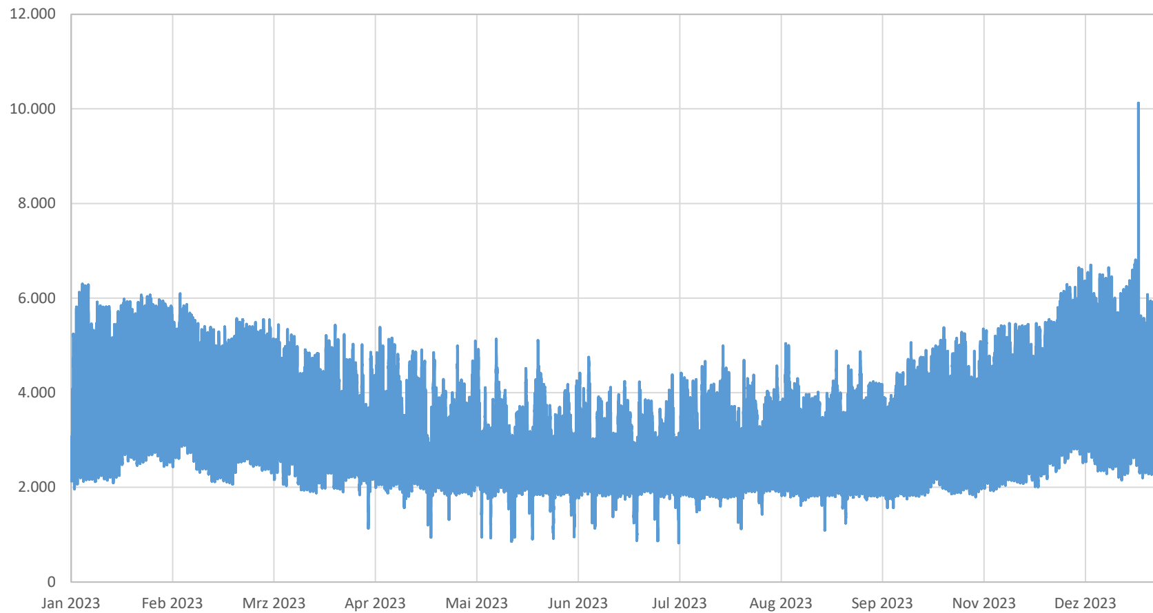
Umspannung MS/NS - Lastverlauf Entnahme vorgelagertes Netz MS (in kW)
