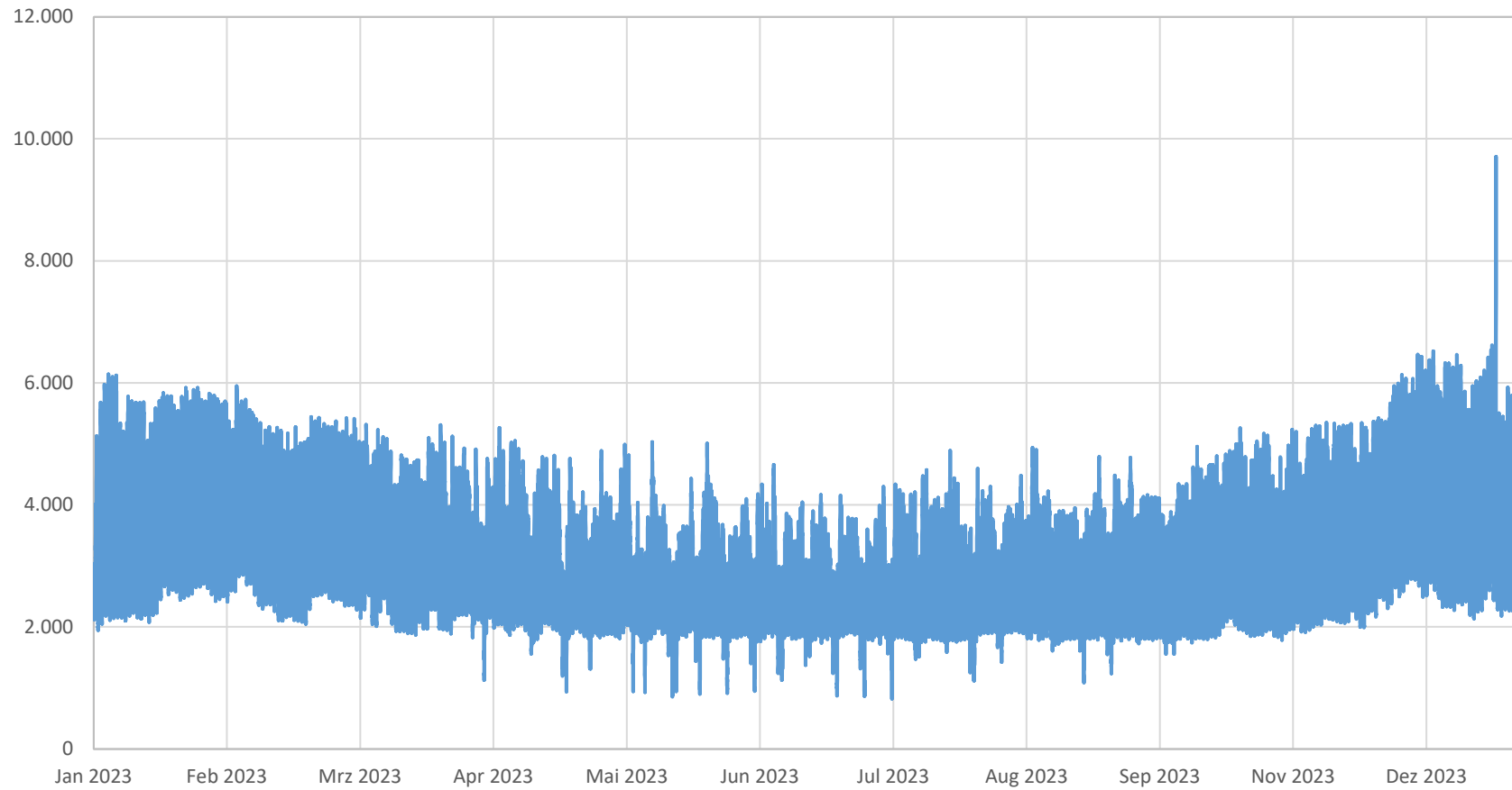
Lastverlauf Umspannung MS/NS (in kW)
