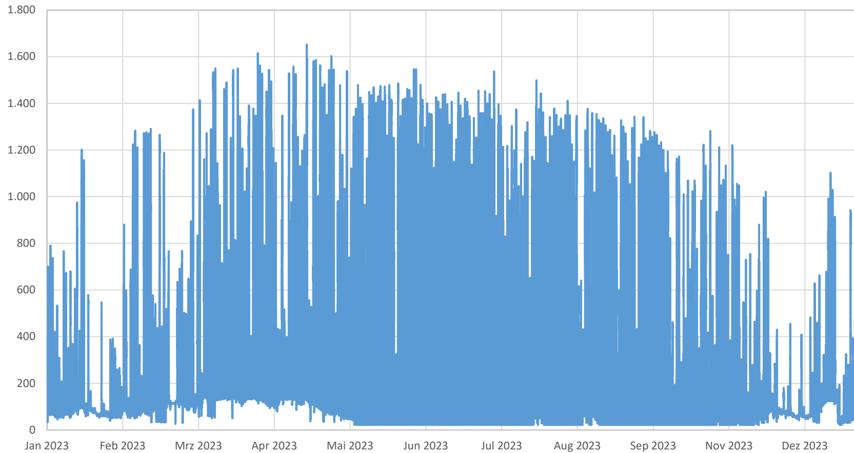
Lastverlauf Einspeisungen Einspeiseanlagen NS (in kW)
