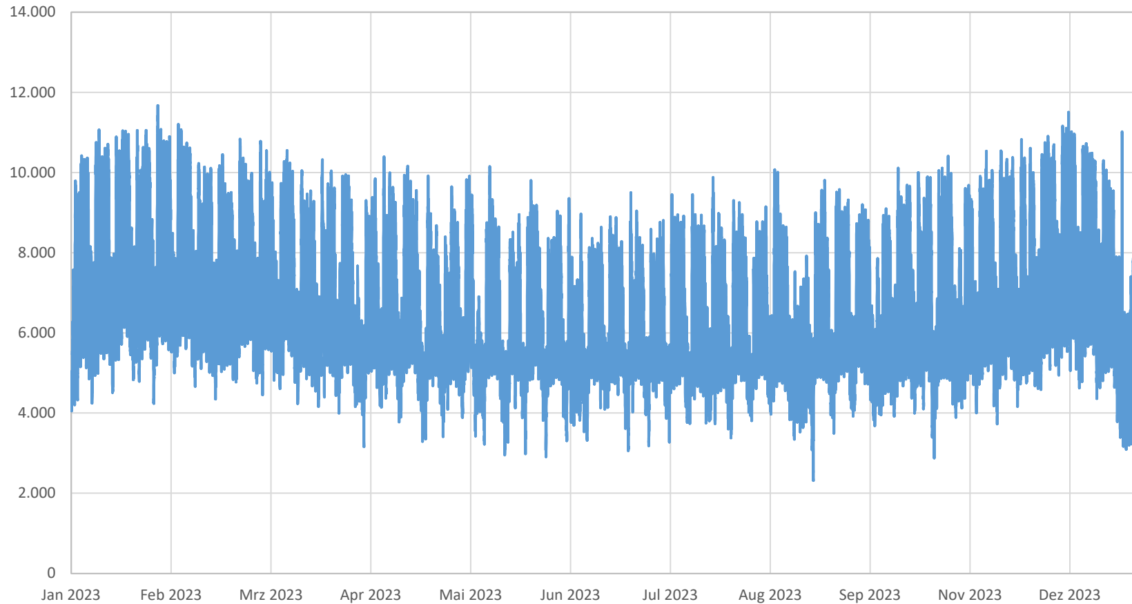
Lastverlauf Mittelspannungsnetz (in kW)
