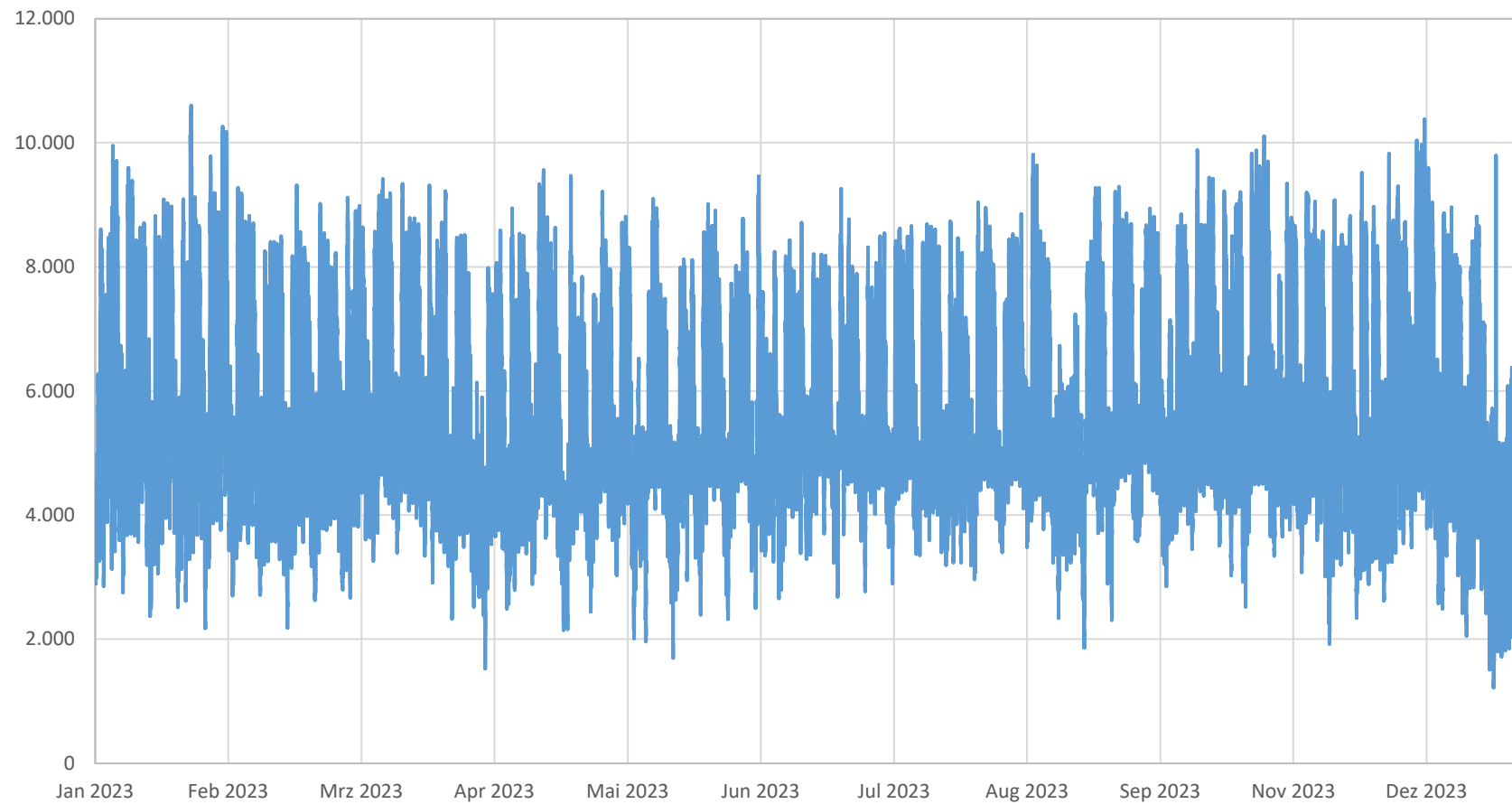
Mittelspannung - Lastverlauf Entnahme vorgelagertes Netz HS/MS und MS (in kW)
