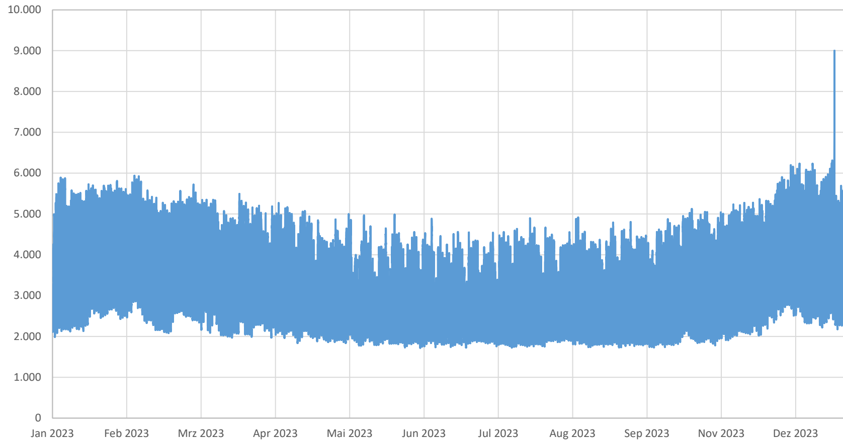
Lastverlauf Niederspannungsnetz (in kW)
