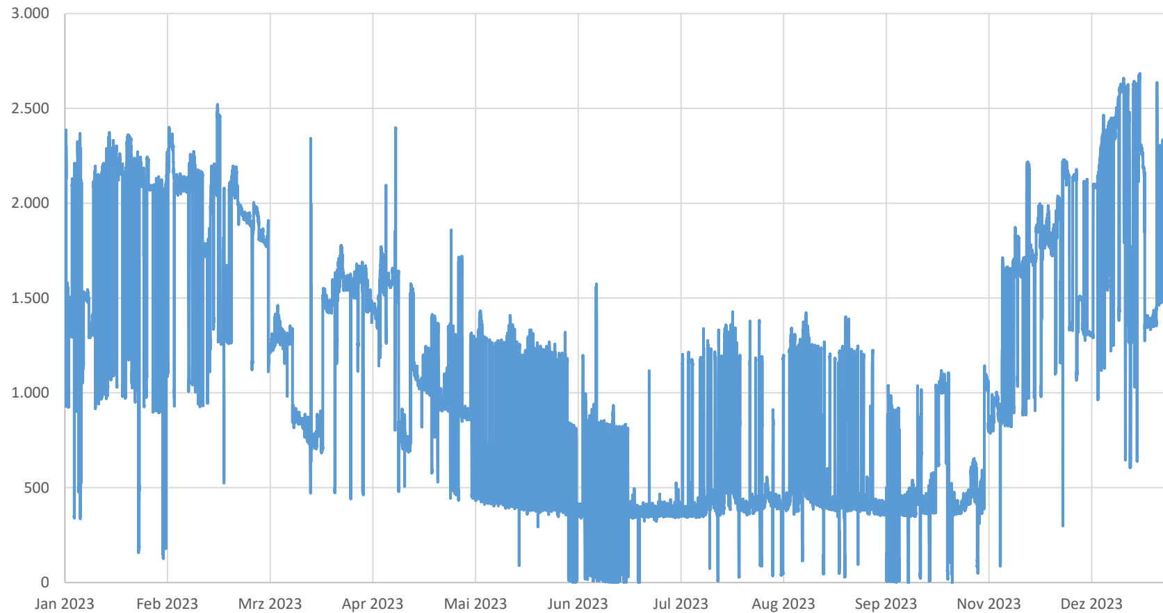
Lastverlauf Einspeisungen Einspeiseanlagen MS (in kW)
