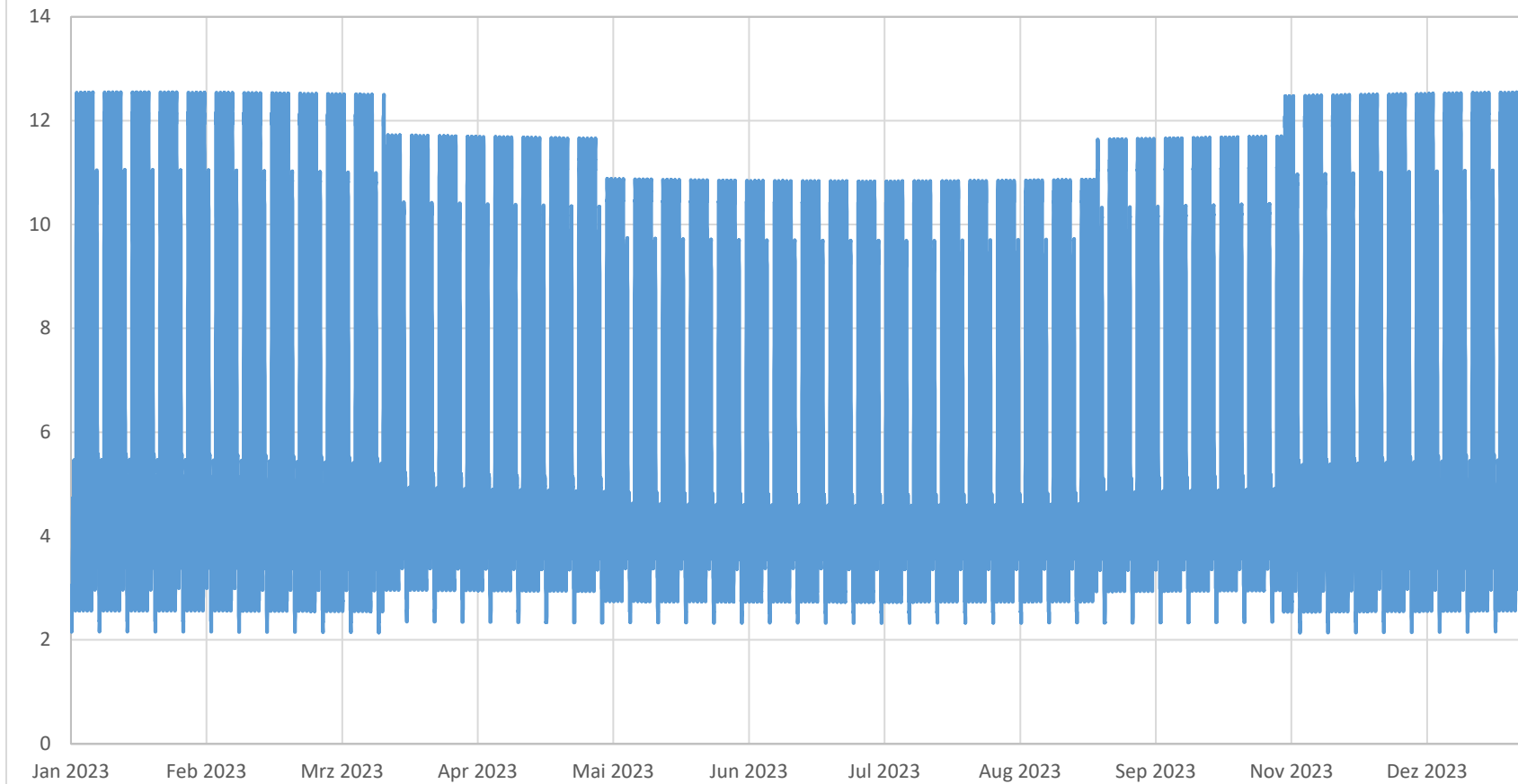
Lastverlauf Entnahme SLP-Kunden - MS (in kW)
