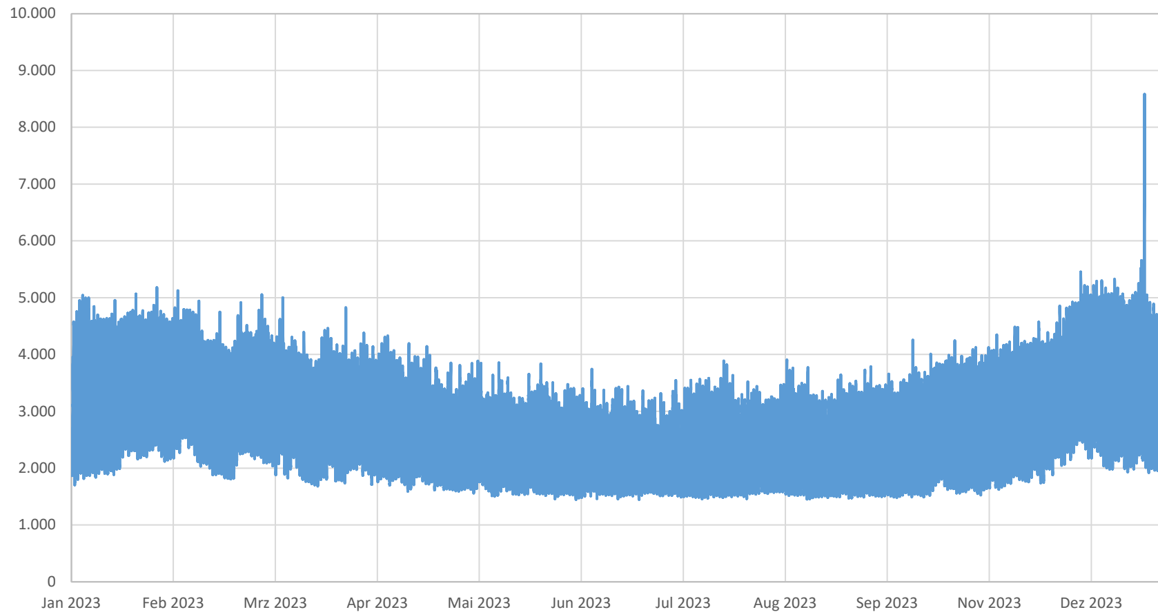
Lastverlauf Entnahme SLP-Kunden - NS (in kW)
