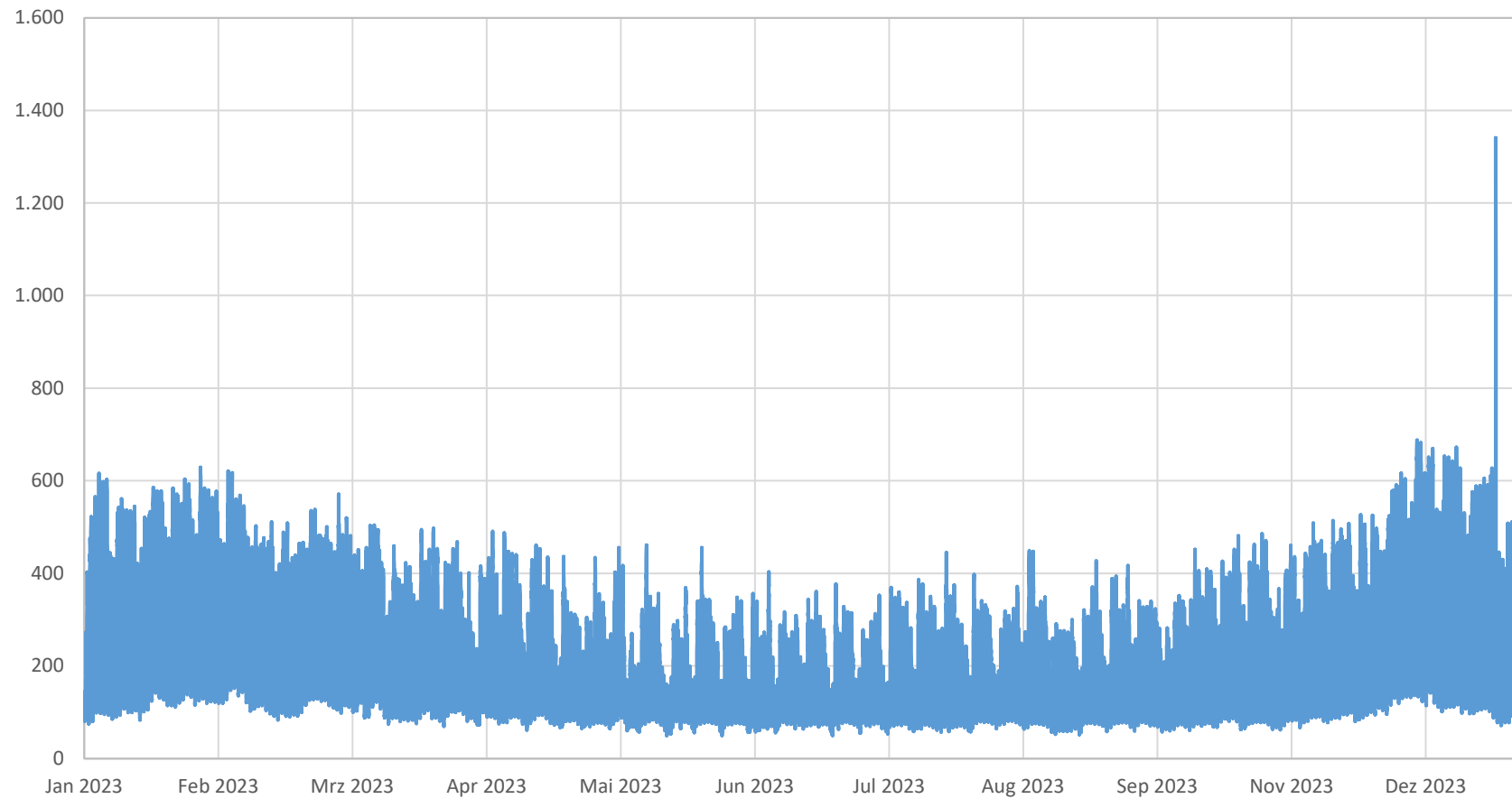
Lastverlauf Netzverluste (in kW)
