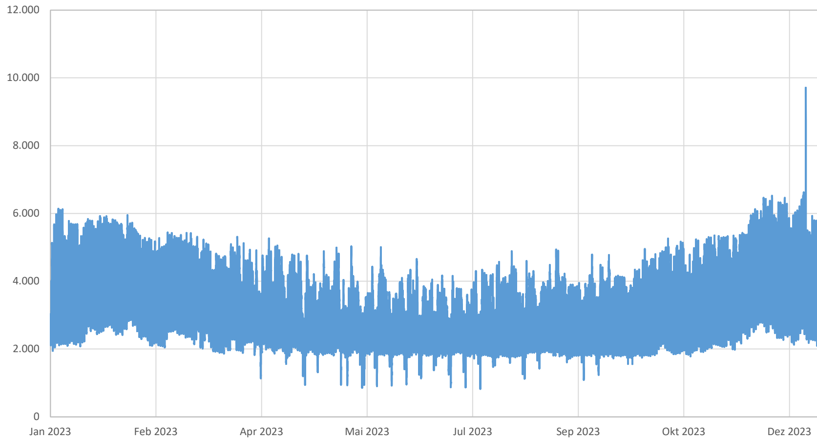
Niederspannung- Lastverlauf Entnahme vorgelagertes Netz MS/NS (in kW)
